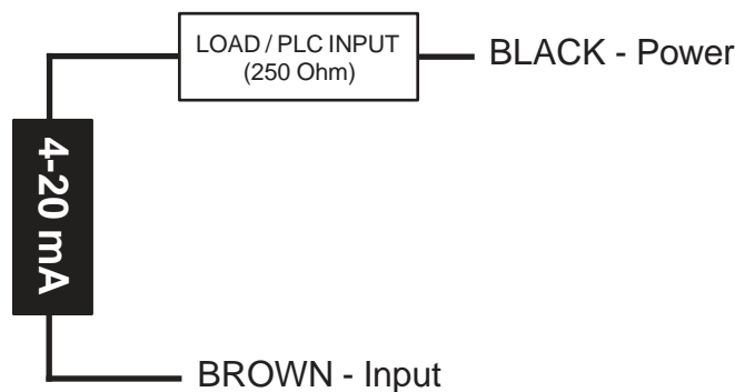
4-20 mA WIRING
