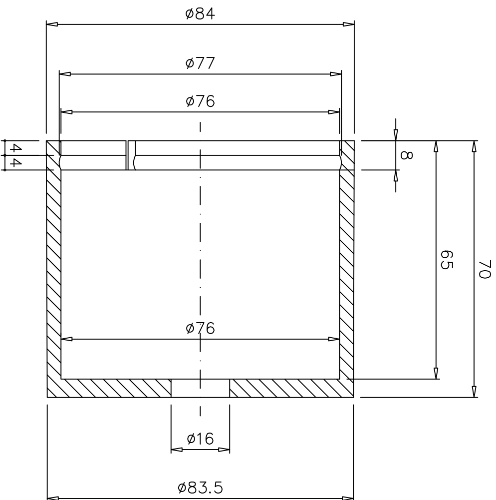
Sez. A-A
