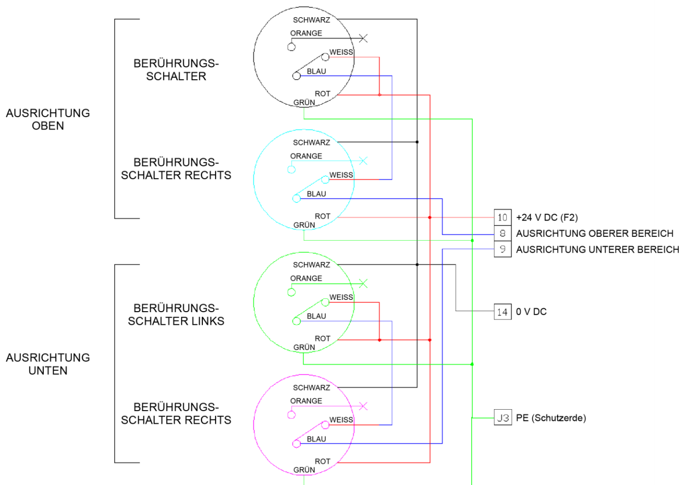
Abbildung 10- TouchSwitch™ Schaltplan
