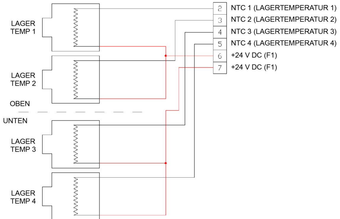
Abbildung 12 – HBS Schaltplan
