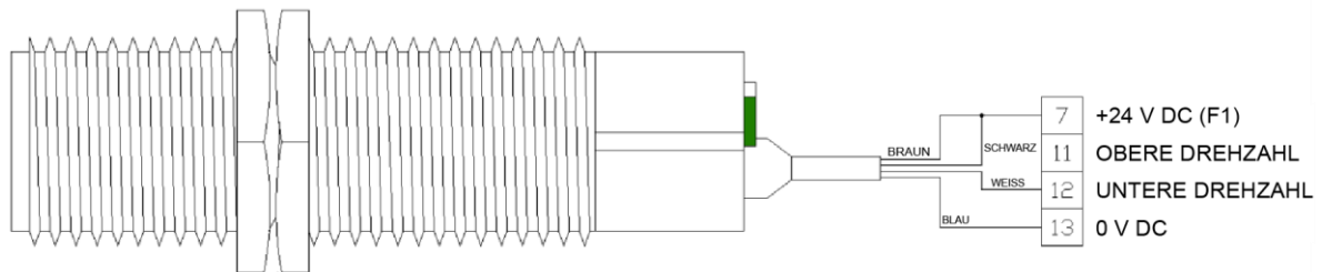
Abbildung 11 – Schaltplan Induktivsensor
